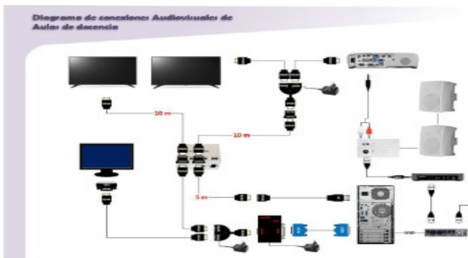
Esquema físico de la conexión de los dispositivos audiovisuales en las aulas de docencia
